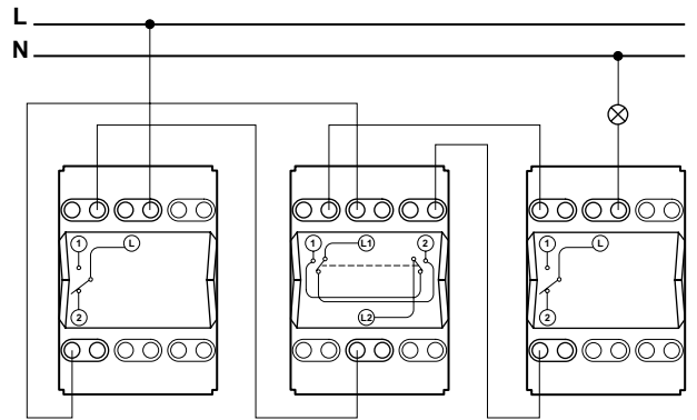
2 выключателя на два направления + 1 промежуточный выключатель
