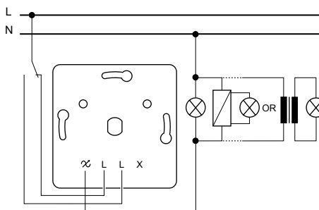
Переключатель - S5xx515
